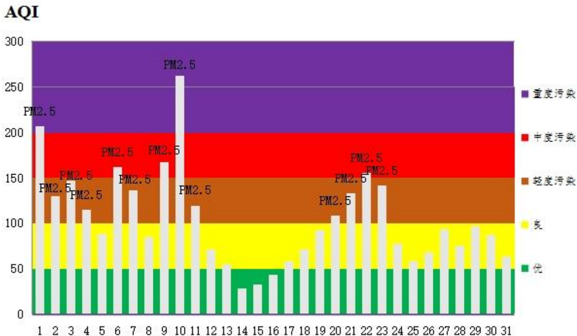
图 2 2023 年 1 月鄂州市区空气质量指数分布图
