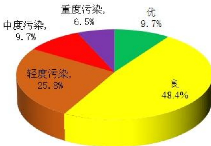
图 2 2023 年 1 月鄂州市区空气质量指数分布图
