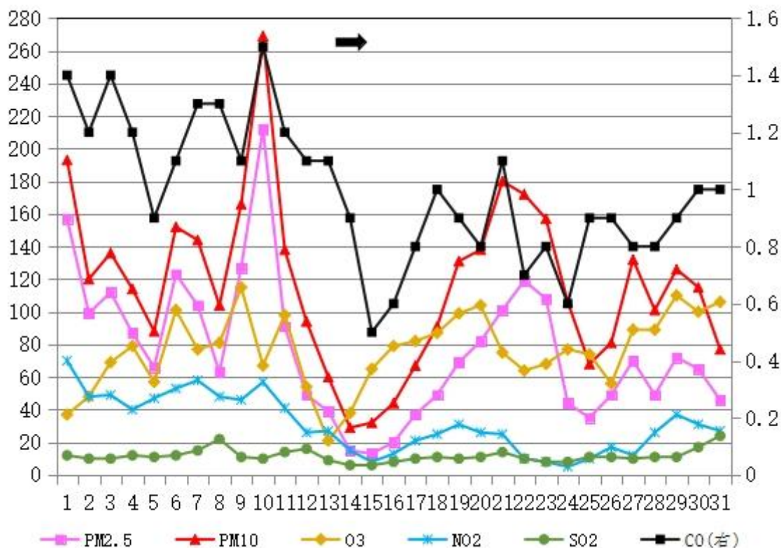
图1 1月份鄂州市城区六项污染物日浓度变化趋势
